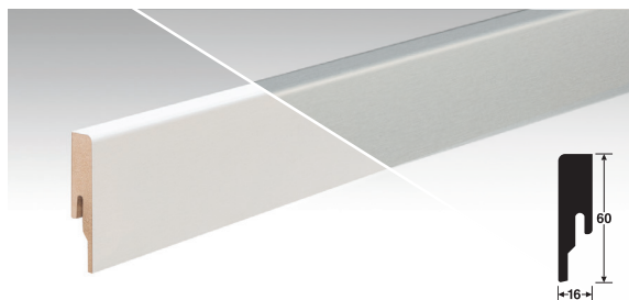
Rodapié acentuado ASL 60 (blanco, a juego, acero inoxidable, antracita, negro) 16 x 60 x 2380 mm
