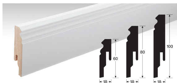
Rodapié Hamburgo HSL 60 | 80 | 100 (blanco) 18 x 60 x 2380 mm 18 x 80 x 2380 mm 18 x 100 x 2380 mm
